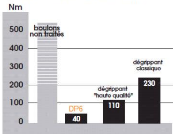
Test MIL A 907 - E/D : couple de desserrage
